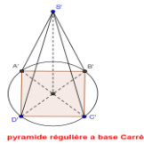
pyramide régulière à base Carré
